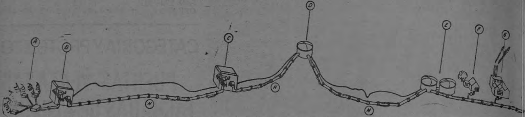
Dibujo que muestra el perfil del nuevo acueducto de Puente de Mulas. Este dibujo se explica así: A) Fuentes; B) Estación de bombeo Nº 1; C) Estación de bombeo Nº 2; D) Tanque de almacenamiento de Bello Horizonte; E) Tanques del Sur; F) Usuarios; G) Industrias; H) Tubería de conducción.
